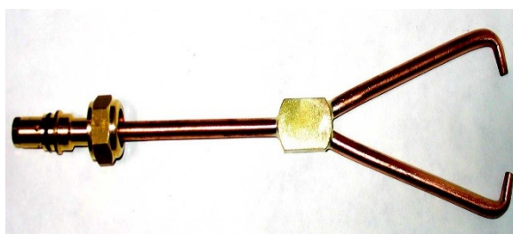
5. Горелка V-формы двухфакельная для метана и пропана ES-MP124
