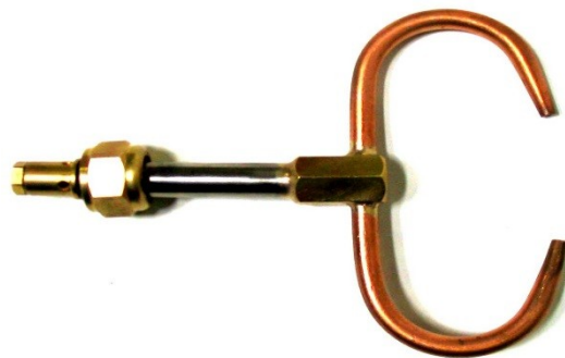
8. Горелка однофакельная для ацетилена ES-A127
